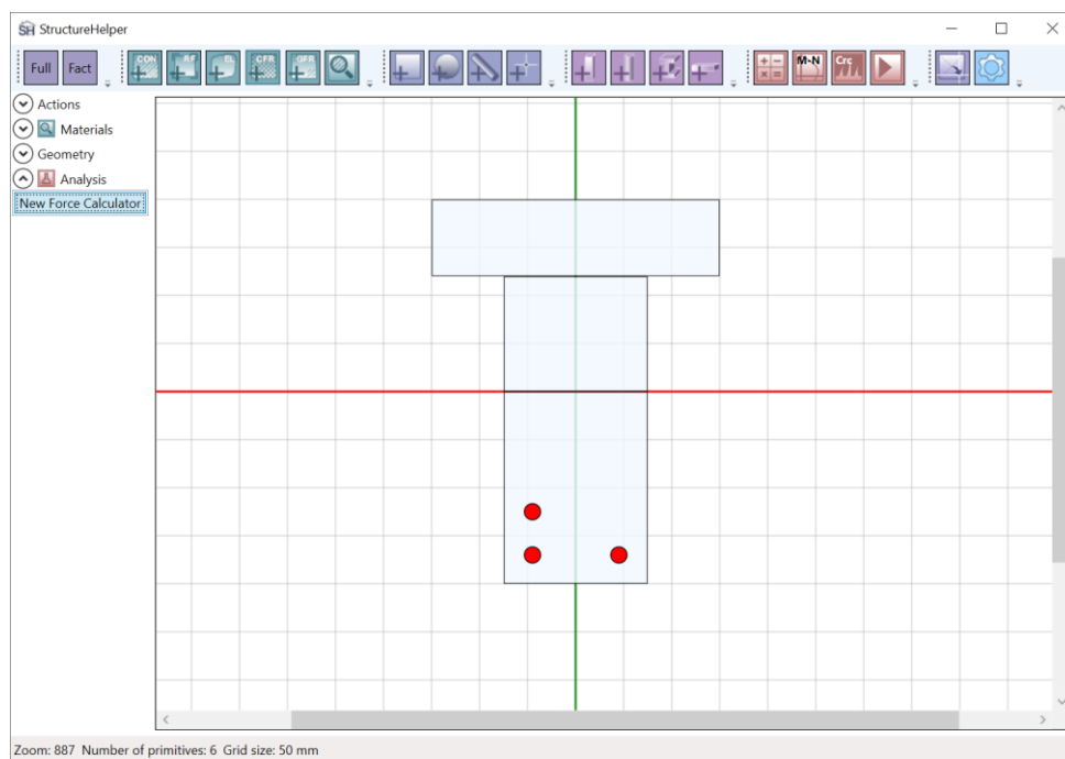
Рисунок 3-10. Расчетное сечение элемента
