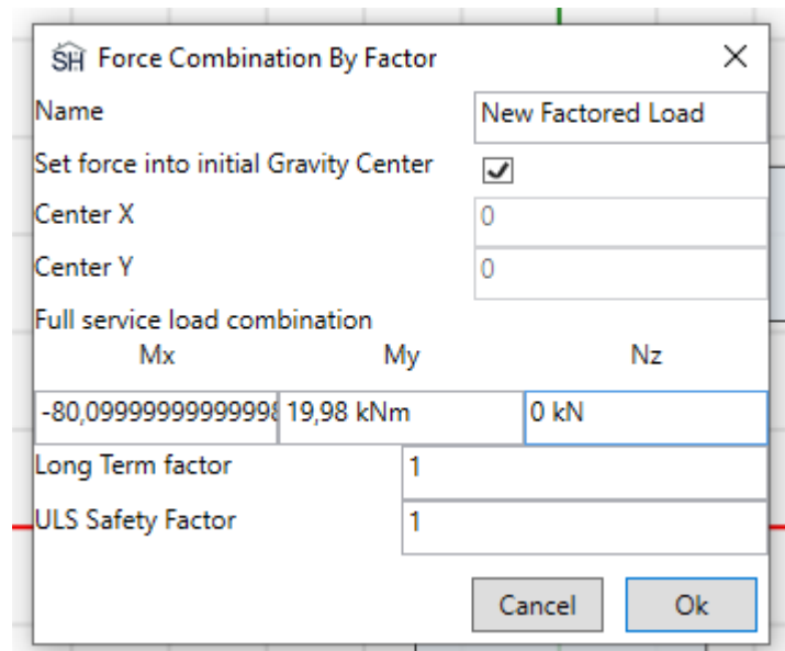
Рисунок 3-14. Свойства загрузки с учетом наклона прогона относительно расчетных осей По результатам выполненного расчета прочность принятого сечения не обеспечена.
