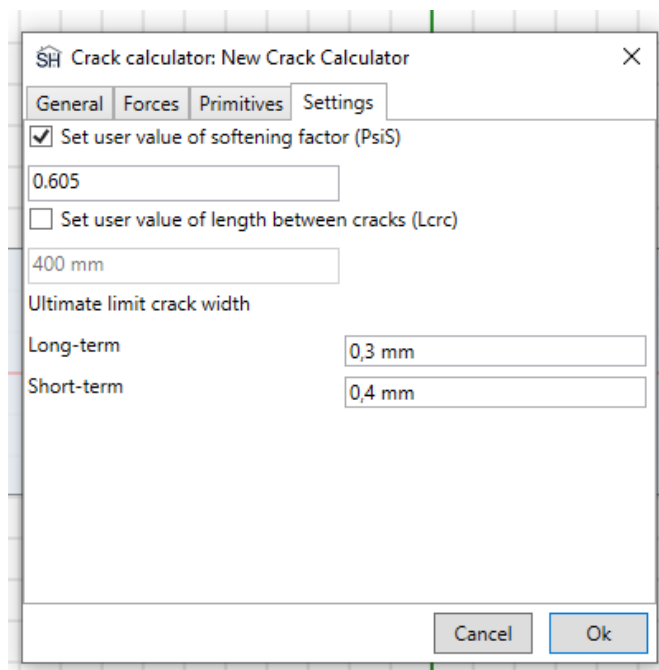
Рисунок 4.2 –учет факторов \psi_s = 0,605 как в пособии
