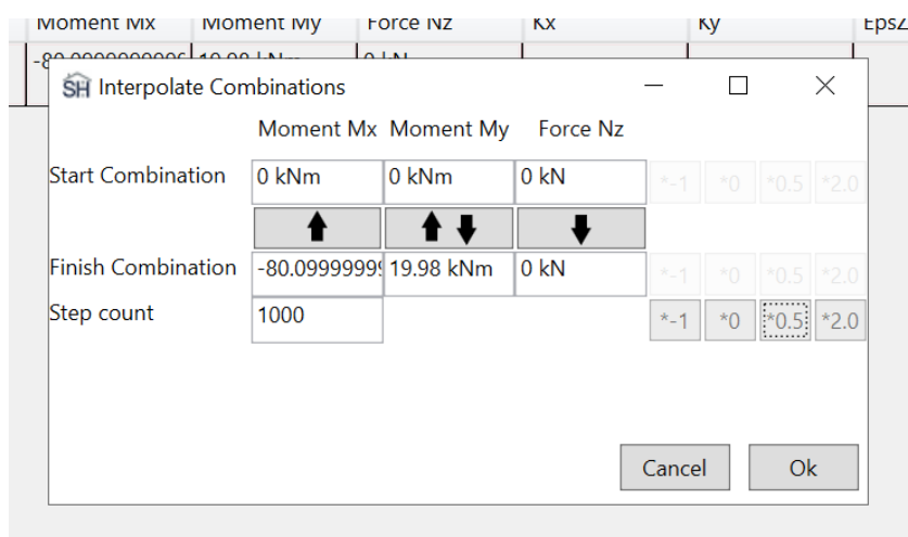
Рисунок 3-16. Условия интерполяции усилий для нахождения предельного момента
