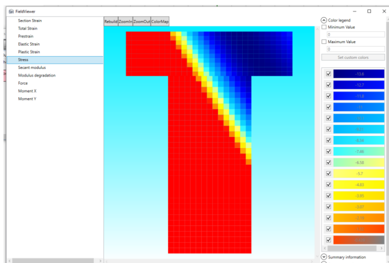
Рисунок 3-19. Изополе напряжений в сечении для примитивов бетона Сравнение результатов расчета
