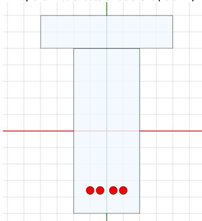
Рисунок 3-2. Расчетное сечение элемента (StructureHelper)
