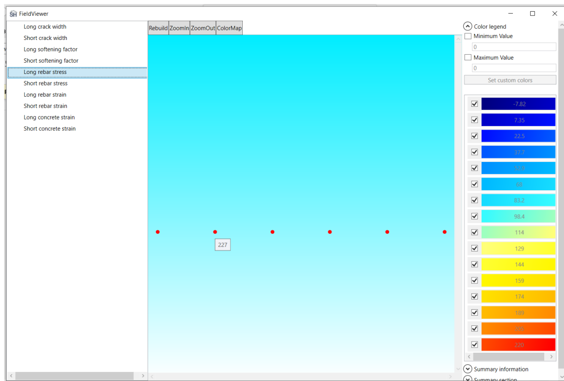
Рисунок 6 – Напряжение в растянутой арматуре
