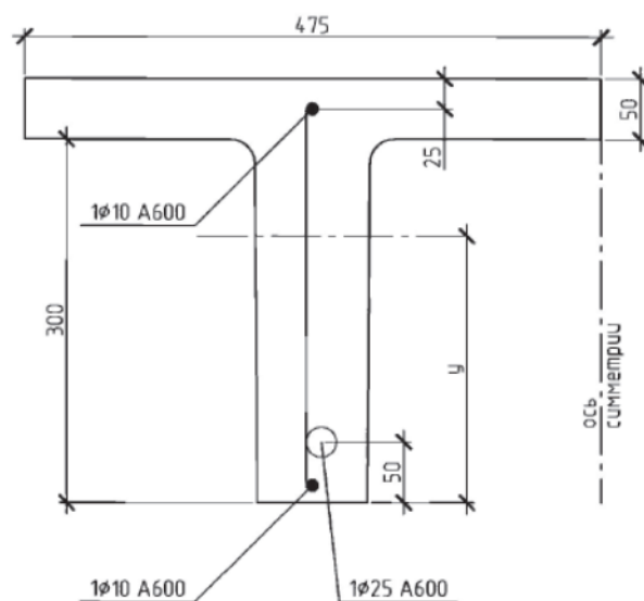
Рисунок 4-9. Поперечное сечение ребристой плиты по данным источника Ввод исходных данных в StructureHelper
