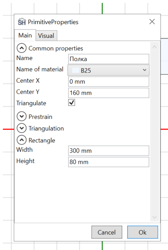
Рисунок 3-13. Свойства примитива для полки толщиной 80мм Зададим комбинацию нагрузок
