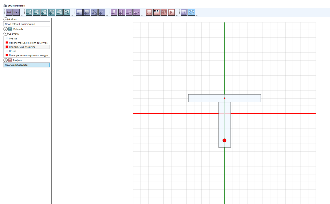
Рисунок 4-10. Поперечное сечение ребристой плиты в программном комплексе StructureHelper
