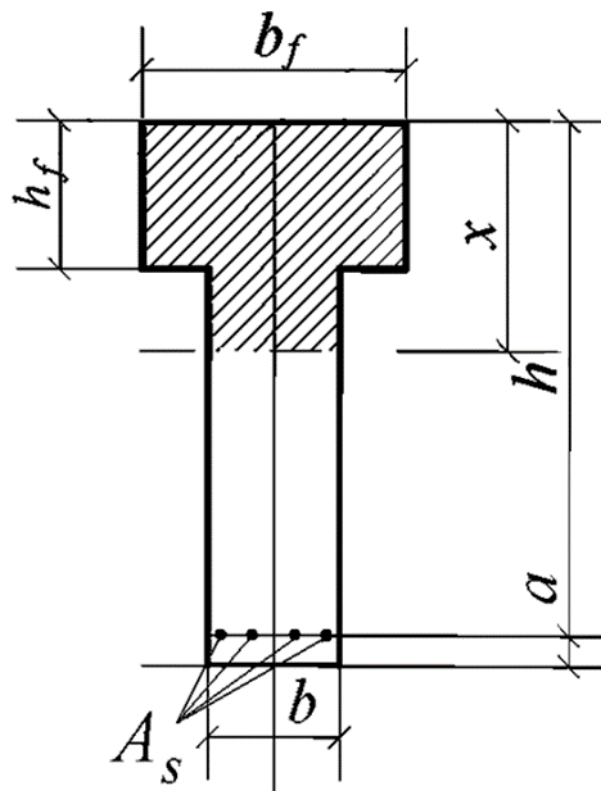
Рисунок 3-1. Расчетное сечение элемента (источник)
