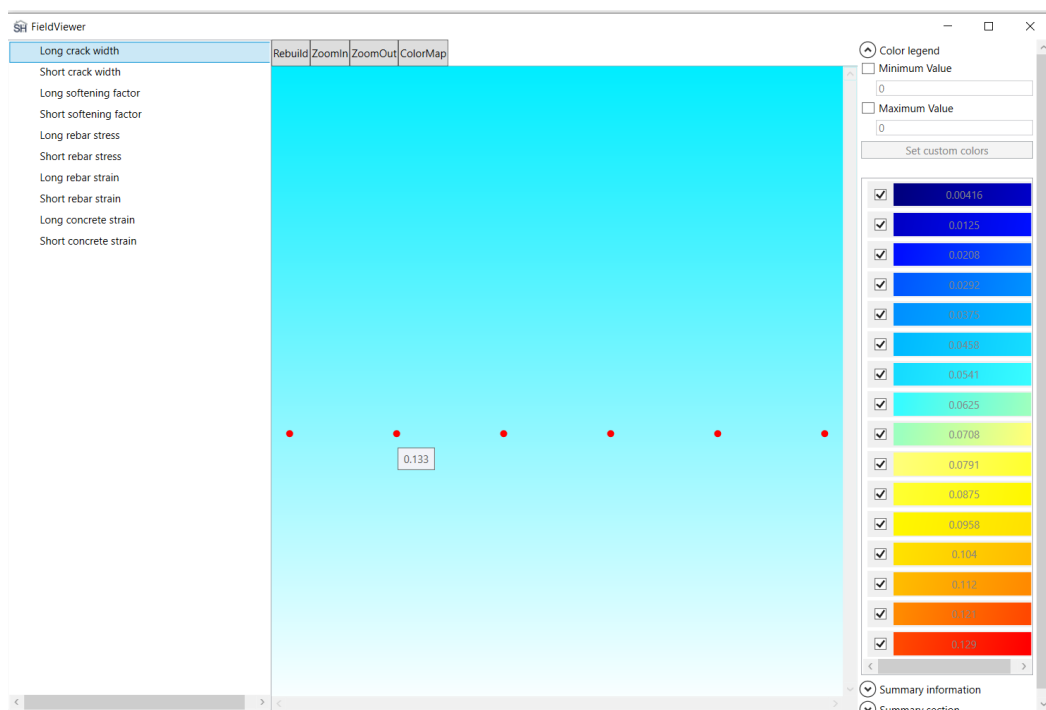
Рисунок 5 – Ширина продолжительного раскрытия трещин
